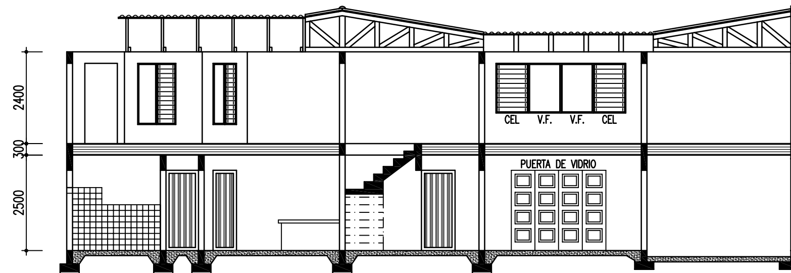
CORTE A-A — 1:100
