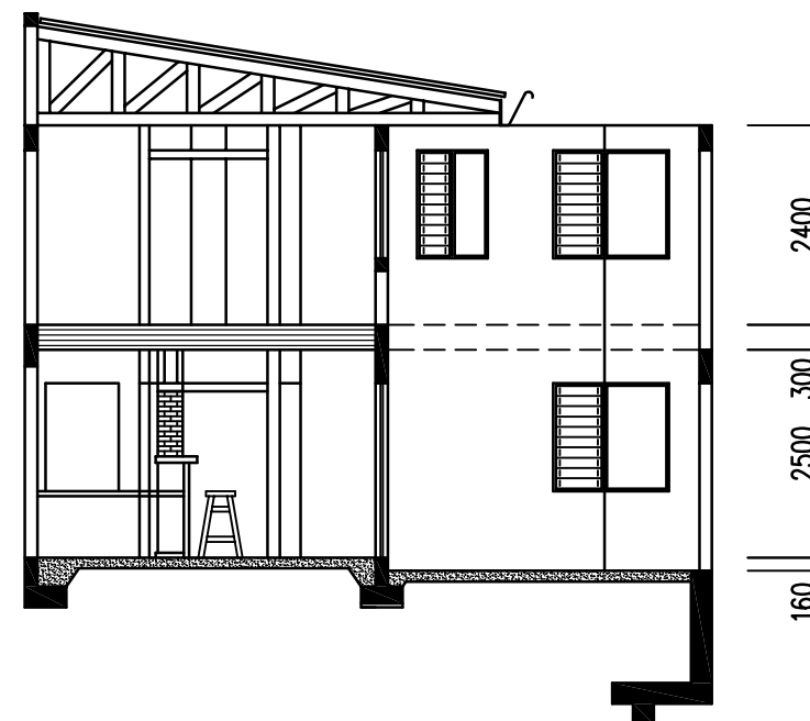
CORTE C-C — 1:100
