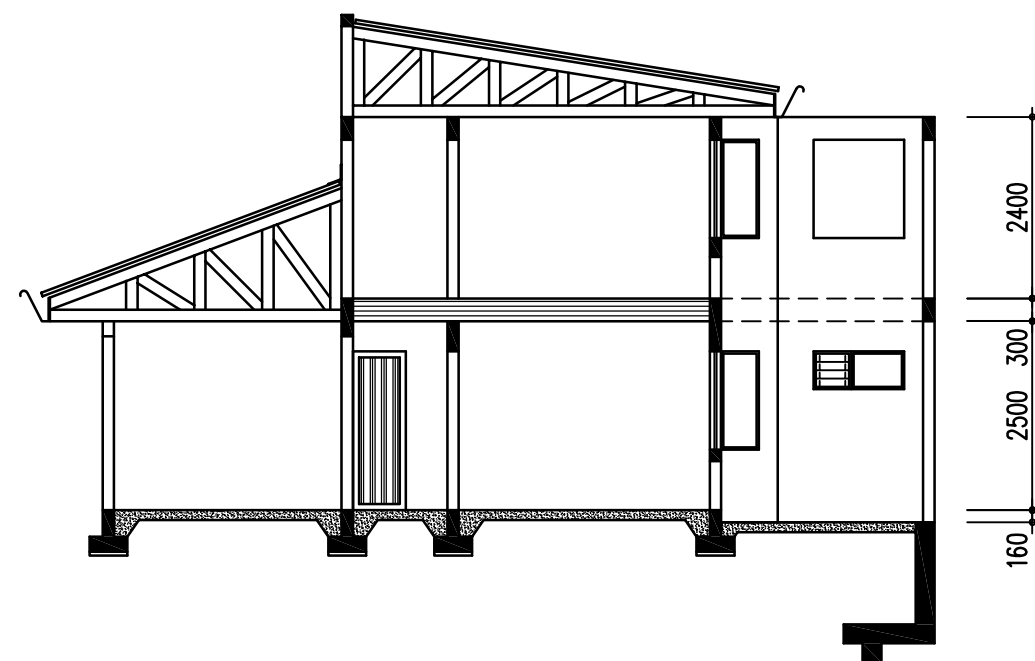
CORTE B-B — 1:100
